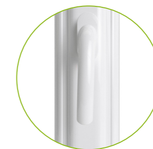
Battement central : 116 mm (vue intérieure)
